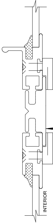
4 MUNTIN DETAIL SCALE: FULL
